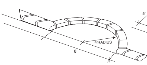
8FT ROMAN END
